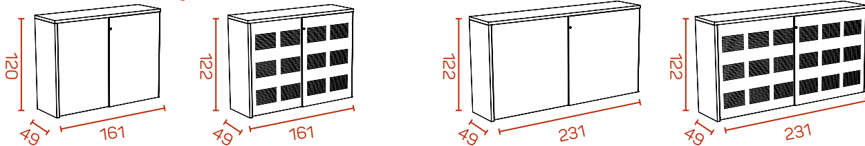
KS-store - luxe uitvoering - aanbouwkasten - 40H
