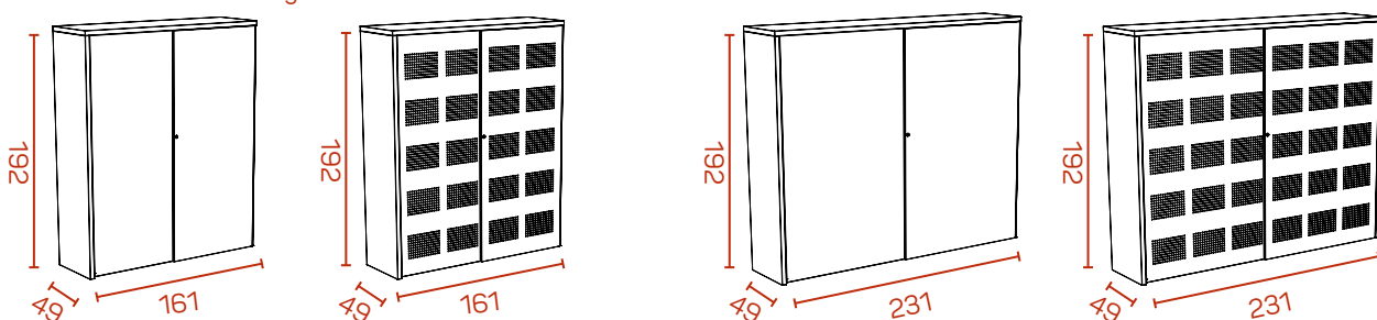
KS-store - luxe uitvoering - aanbouwkasten - 50H
