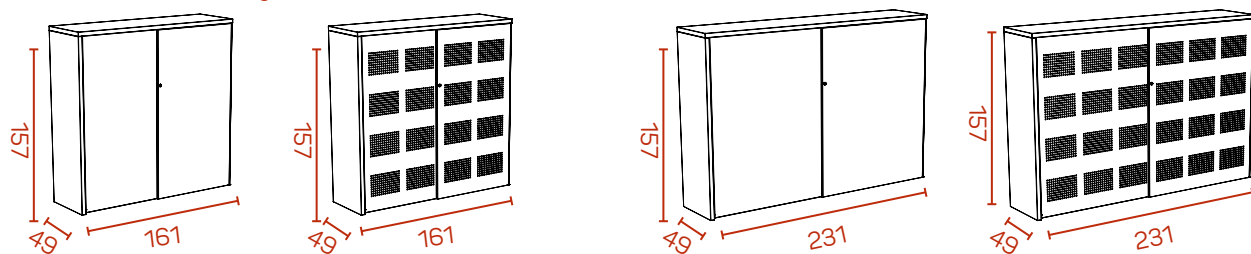
KS-store - luxe uitvoering - aanbouwkasten - 50H
